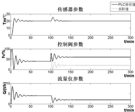
图8 攻击控制阀节点
