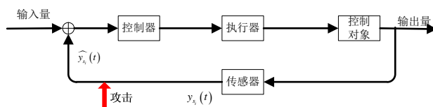
图 3 单回路控制系统
