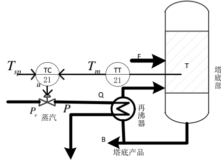
图 5 提馏段温度单回路控制方案
