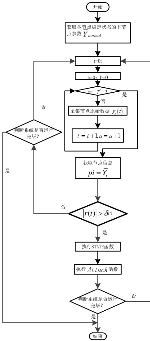
图 4 算法流程图
