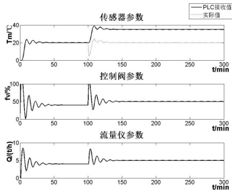
图7 攻击温度传感器
