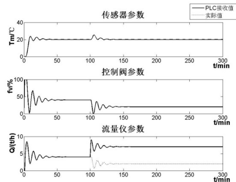
图9 攻击流量仪
